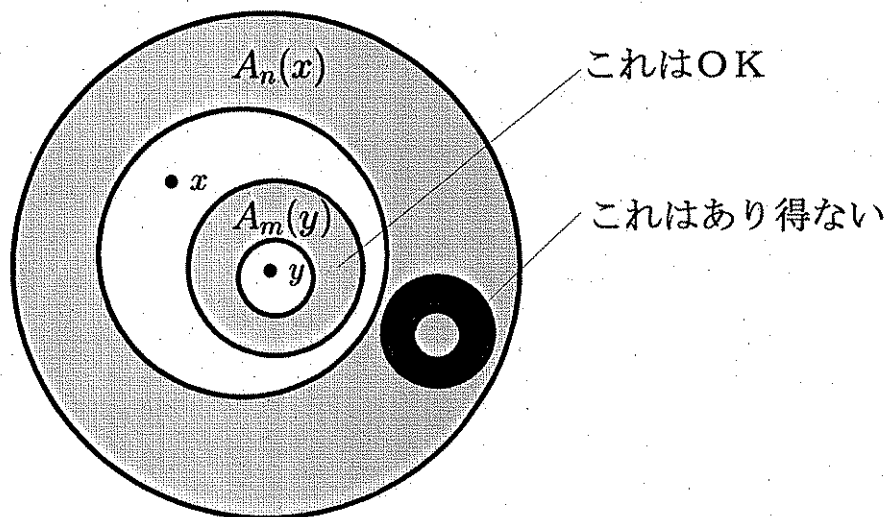
Figure 5.5 A_n(x) と A_m(y) の位置関係.
