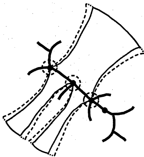
Figure 5.2 Q^{(i)} と U^{(i)} .
